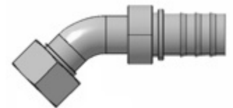
DIN 3863 - 60° / DIN 3865 - 24° Metrische wartel, lichte serie - 45° elleboog Metric swivel, light series - 45° elbow
