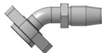
“Bock” flensaansluiting, 45° elleboog “Bock” flange connection, 45° elbow
