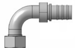
DIN 3863 - 60° Metrische wartel, lichte serie - 90° elleboog Metric swivel, light series - 90° elbow
